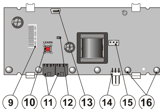
Figure 2: 9 - Code fabricant; 10 - Bouton LEARN (inscription); 11 - Connecteur de la pile; 12 - Indicateur de défaillance jaune; 13 - Connecteur mini USB; 14 - Connexion de la sirène piezo (attention: haute tension); 15 - Connecteur de l'antenne extérieure; 16 - Clignotants à LED rouge à haute intensité
